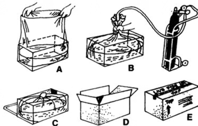
Requerimiento y secuencia del envase de peces por el método de las bolsas de polietileno
